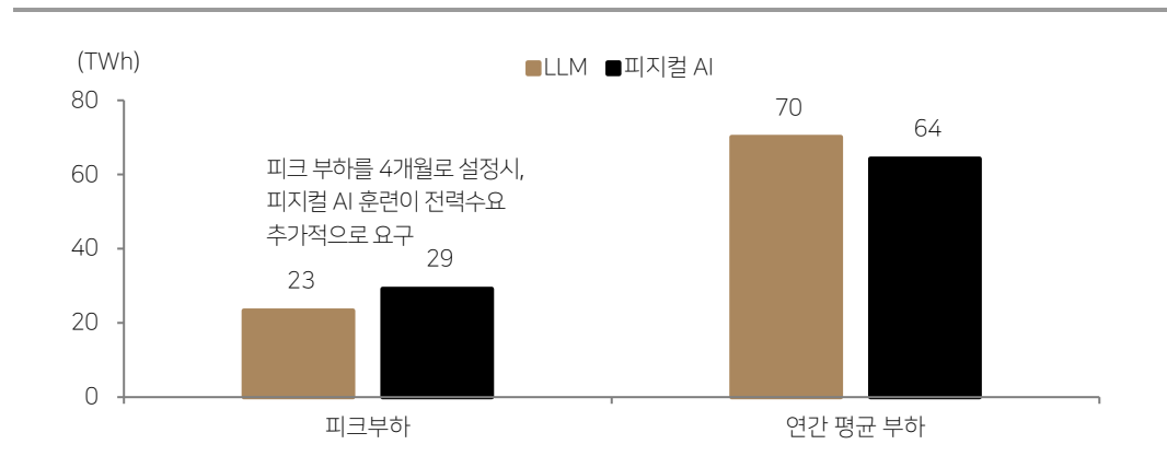
Fig. 23: LLM과 피지컬 AI의 부하 비교
