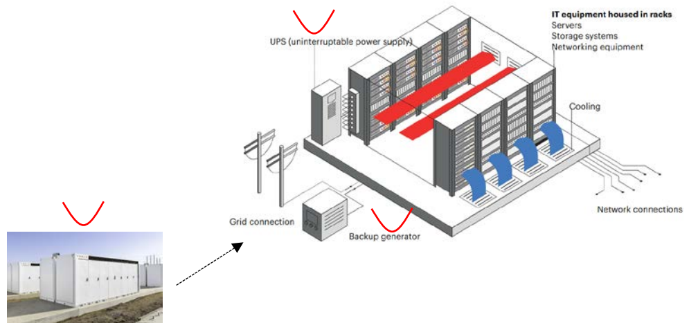
Fig. 32: AI 데이터센터 및 외부 ESS형태: 데이터센터 내부에는 UPS, BBU가, 외부에는 그리드 ESS가 위치해, 서버 부하 증가에 따른 ESS수요 동반
