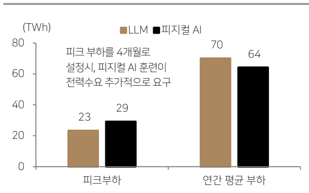
Focus Chart 7 LLM과 피지컬 AI의 부하 비교
