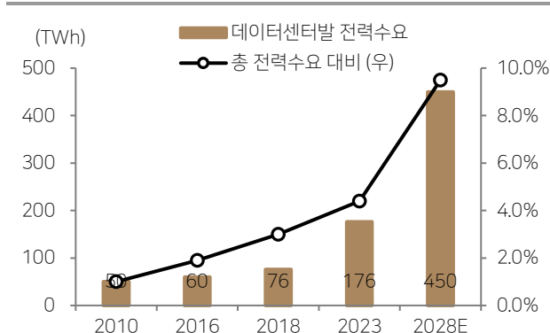
Fig. 1: 미국 데이터센터 전력수요 28년 450TWh 초과가능
