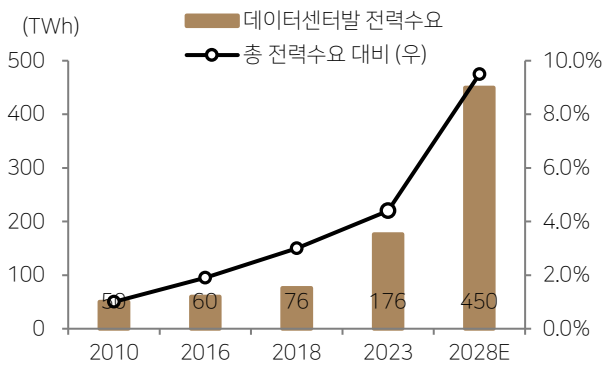
Focus Chart 1 미국 데이터센터 전력수요 28년 450TWh 초과 가능
