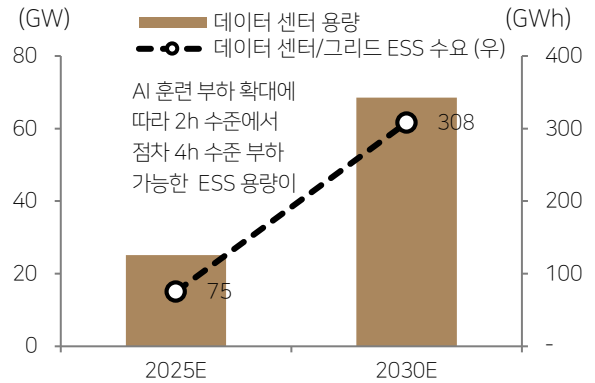
Focus Chart 2 미국 데이터센터/그리드 ESS수요 추정: 300GWh 수준까지도 가능
